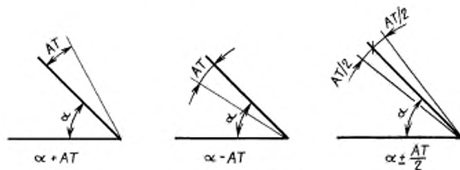
\alpha — номинальный угол Черт. 2
