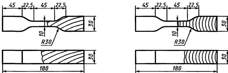
Образцы для определения модуля упругости при растяжении поперек волокон
